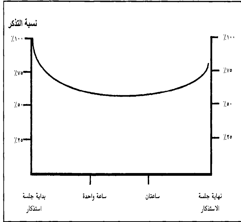
شكل رقم ٤ منحنى التذكر أ.
